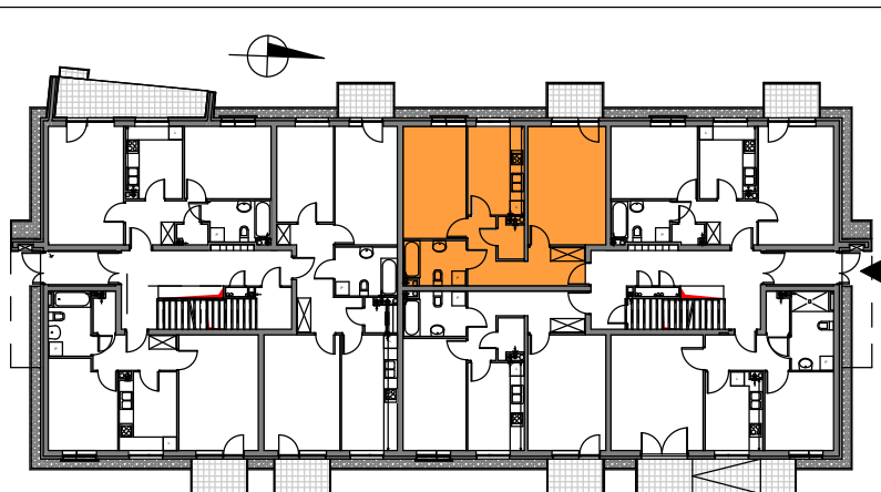
SCHEMAT ROZMIESZCZENIA MIESZKAŃ BUDYNKU nr 3
