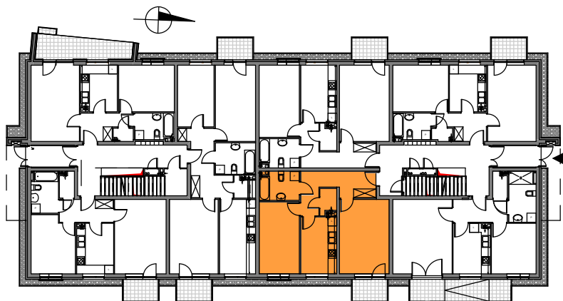
SCHEMAT ROZMIESZCZENIA MIESZKAŃ BUDYNKU nr 3
