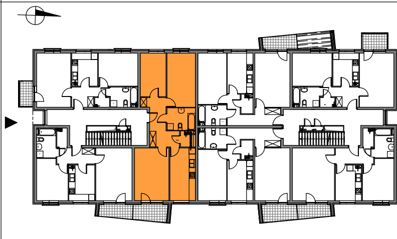
SCHEMAT ROZMIESZCZENIA MIESZKAŃ BUDYNKU NR 7
