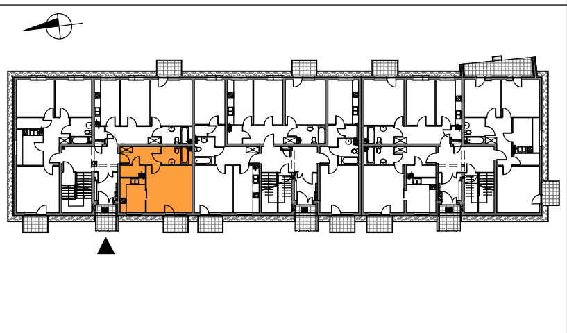
SCHEMAT ROZMIESZCZENIA MIESZKAŃ BUDYNKU NR 1
