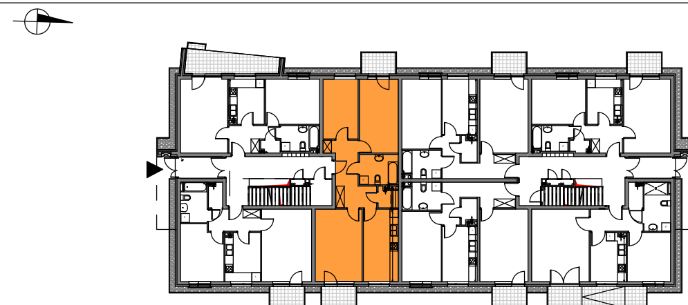
SCHEMAT ROZMIESZCZENIA MIESZKAŃ BUDYNKU nr 7
